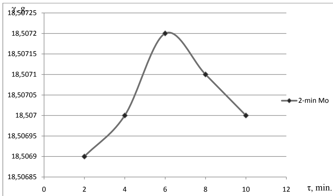
Fig. 2.4 Variația masei catodului din oțel inox la alierea prin scânteii.
