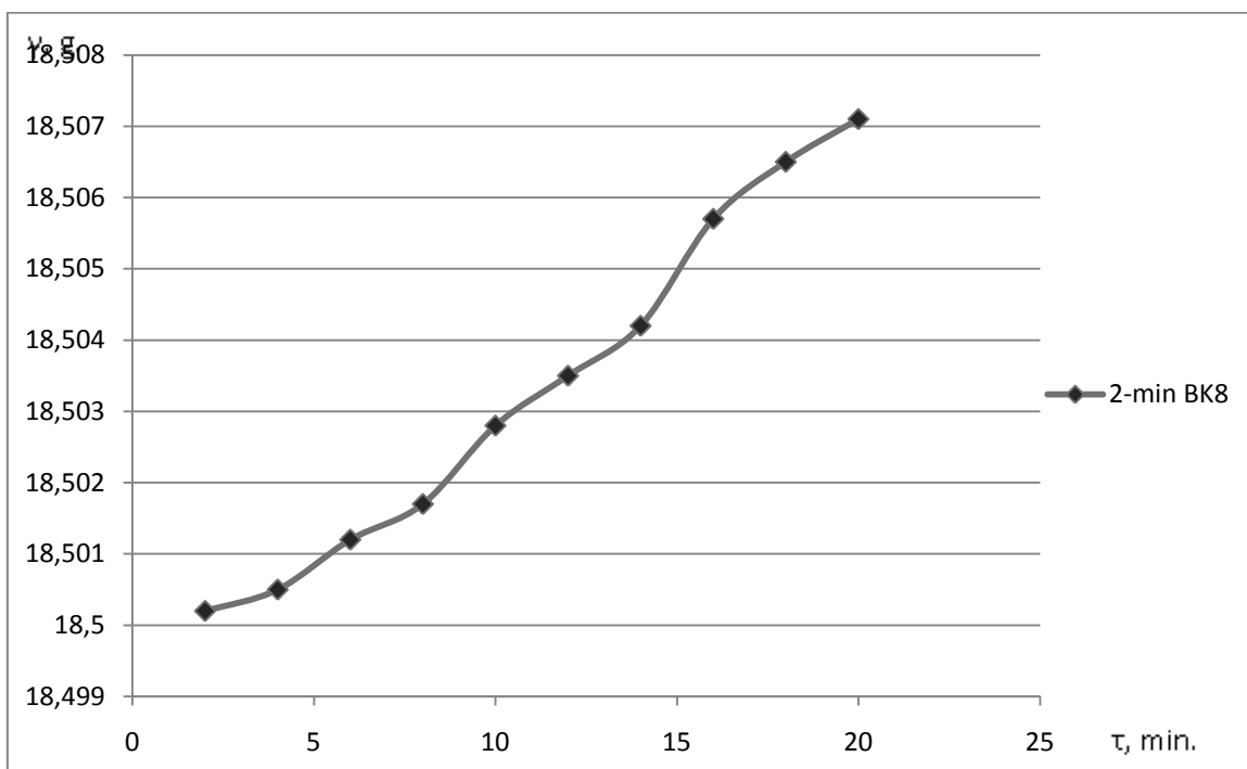
Fig. 2.3 Variația masei catodului din oțel inox la alierea prin scânteii .
