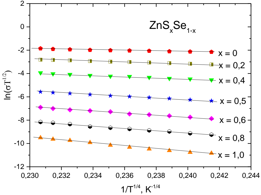
Fig. 3. Dependențele de tip \ln(\sigma T^{1/2}) = f(T^{-1/4}) ale straturilor subțiri de ZnS_xSe_{1-x}
