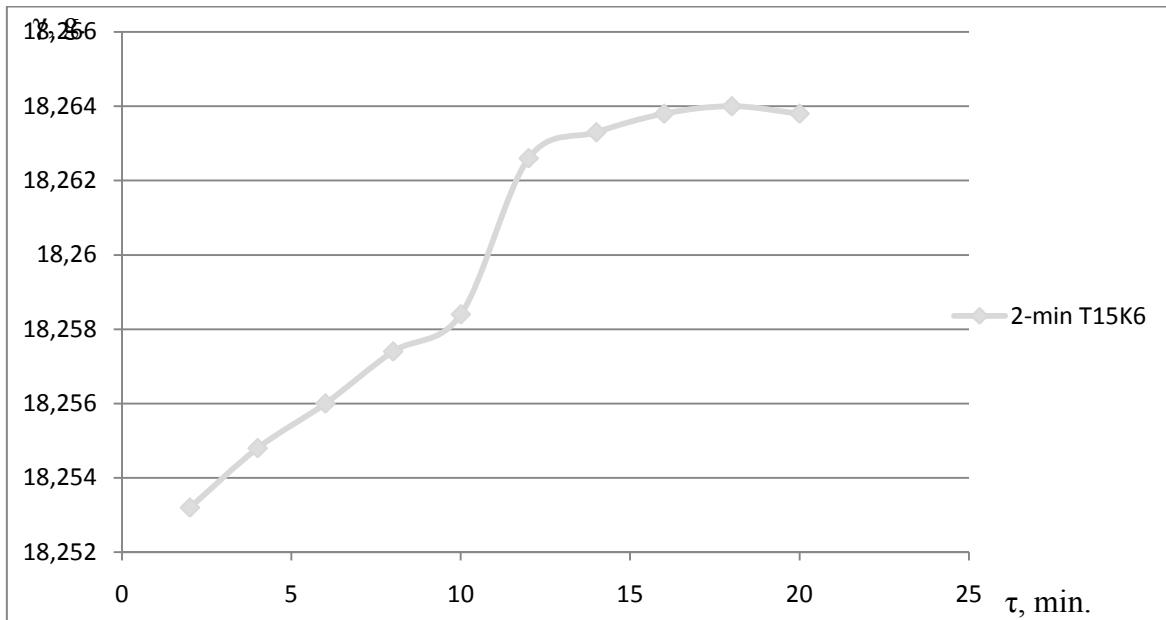
Fig. 2.2 Variația masei catodului din oțel inox la alierea prin scânteii .
