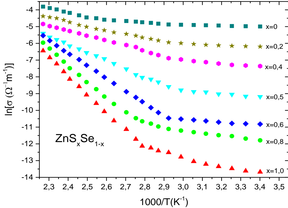
Fig. 1. Dependențele de tip \ln\sigma = f(10^3/T) (II încălzire) pentru straturile subțiri de ZnS_xSe_{1-x} .
