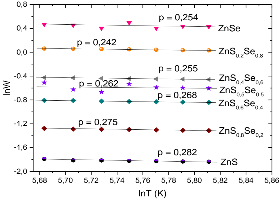
Fig. 2. Dependentele de tip \ln W=f(\ln T) pentru straturile subțiri de ZnS_xSe_{1-x} . Logaritmăm ultima relație, apoi diferențiem relația obținută și după mai multe transformări, obținem:
