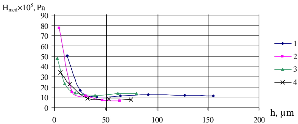
Fig.5 Dependenta valorii microdurității de adâncimea stratului superficial a pieselor executate din Oțel 45 după interacțiunea descărcărilor electrice în impuls pentru: C=8μF; f=8Hz; V=1mm/s; S=0,5mm; 1- W=0,26J, n=2 treceri; 2-W=0,42J, n=2 treceri; 3-W=0,58J, n=2 treceri; 4-W=0,26J, n=3 treceri; electrodul sculă-catod.
