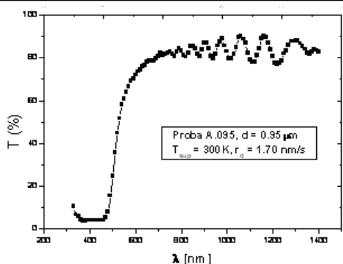
Fig. 9. Dependența T = f(\lambda) pentru proba A.095.
