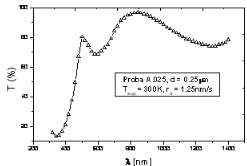
Fig. 4. Dependenta T = f(\lambda) pentru proba A.025.
