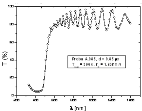
Fig. 8. Dependenta T = f(\lambda) pentru proba A.085.
