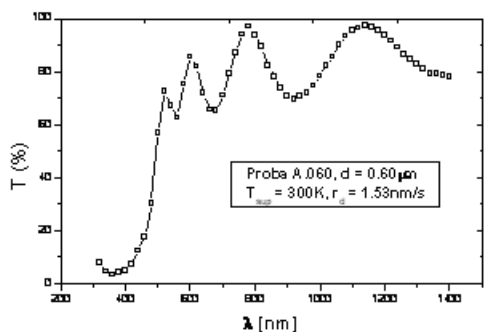
Fig. 6. Dependenta T = f(\lambda) pentru proba A.060.
