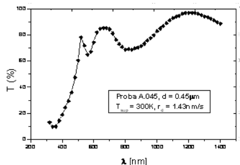
Fig. 5. Dependenta T = f(\lambda) pentru proba A.045.
