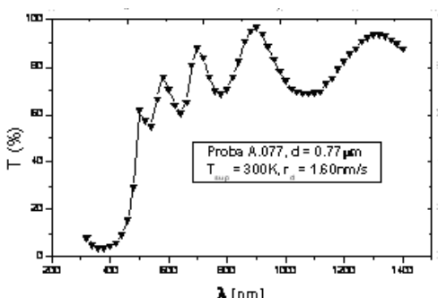
Fig. 7. Dependenta T = f(\lambda) pentru proba A.077.
