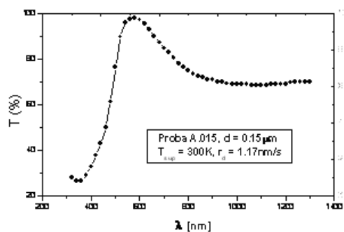
Fig. 3. Dependenta T = f(\lambda) pentru proba A.015.
